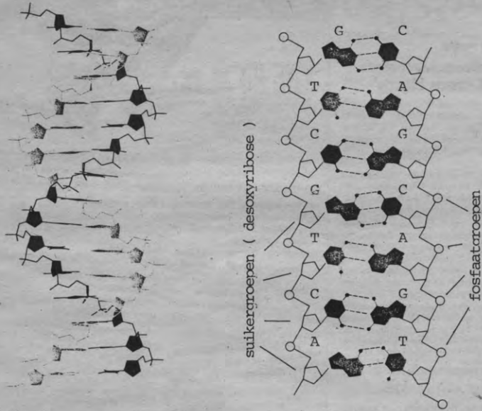
Fig. 1: Model van de DNA-dubbel-helix. De diameter van de helix bedraagt ongeveer 20 Å
