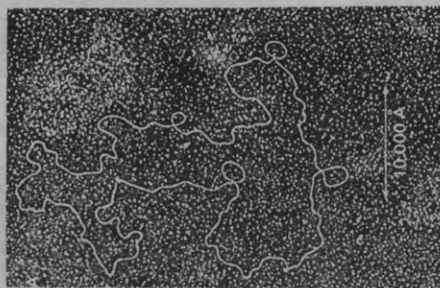
Fig. 3 & 4: Opname van DNA-moleculen door een electronenmicroscop
